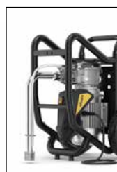
Stijf aanzuigsysteem met stijve retourslang
