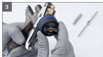
3 Assemblage van de luchtkap
