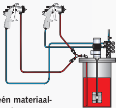
Men kan met één materiaal-drukvat probleemloos twee spuitpistolen met materiaal voeden.
