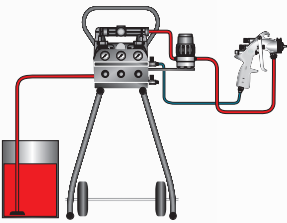
Eerst pompdruk, dan filterdrukregelaar en ten slotte verstuiverdruk instellen. Nu kan het werk beginnen.
