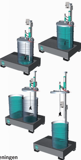
Dekselhefvoorzieningen bestaan ook voor de drukvaten MDG 45 en MDG 60.
